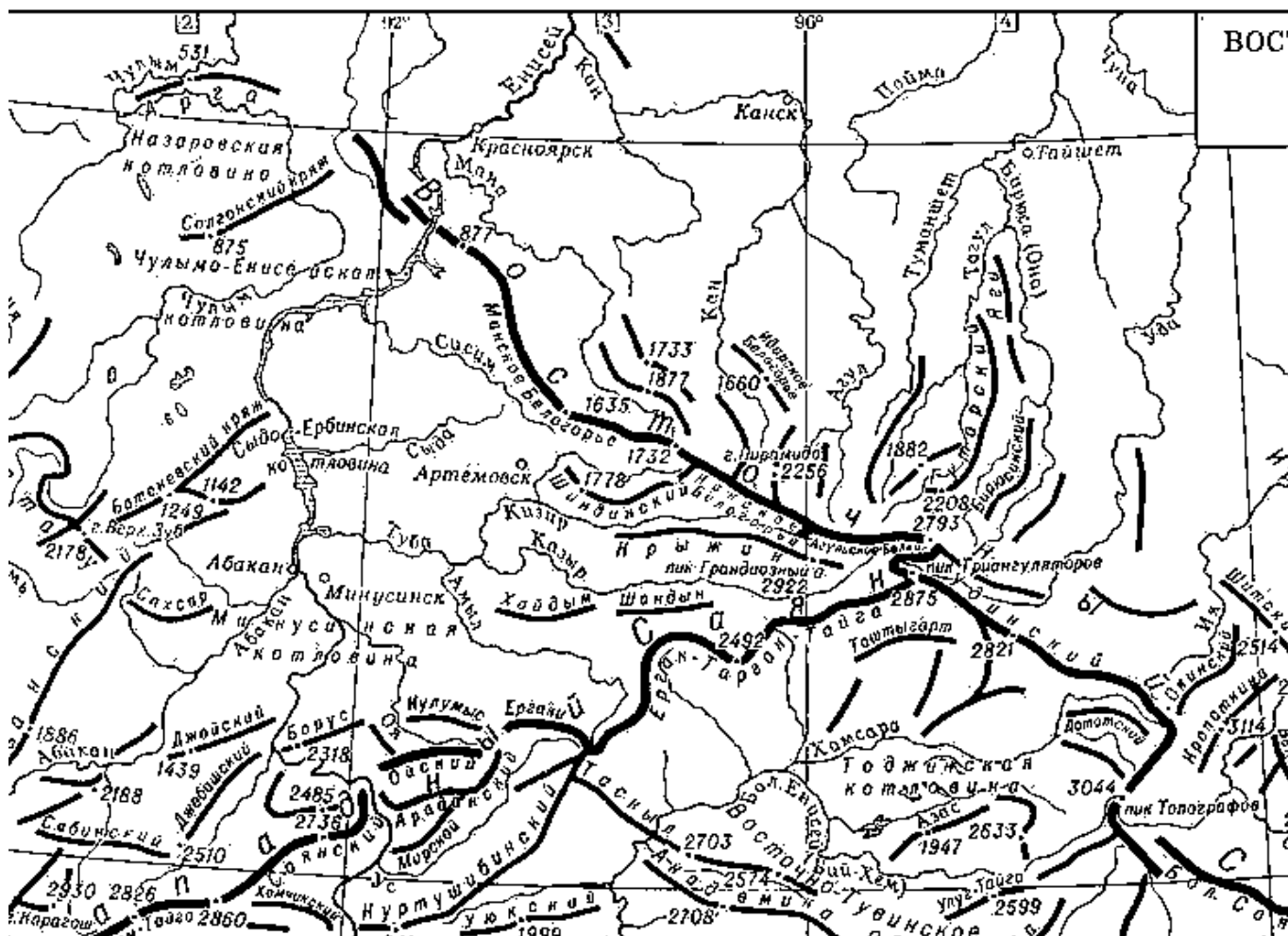
Схема хребтов Саян
